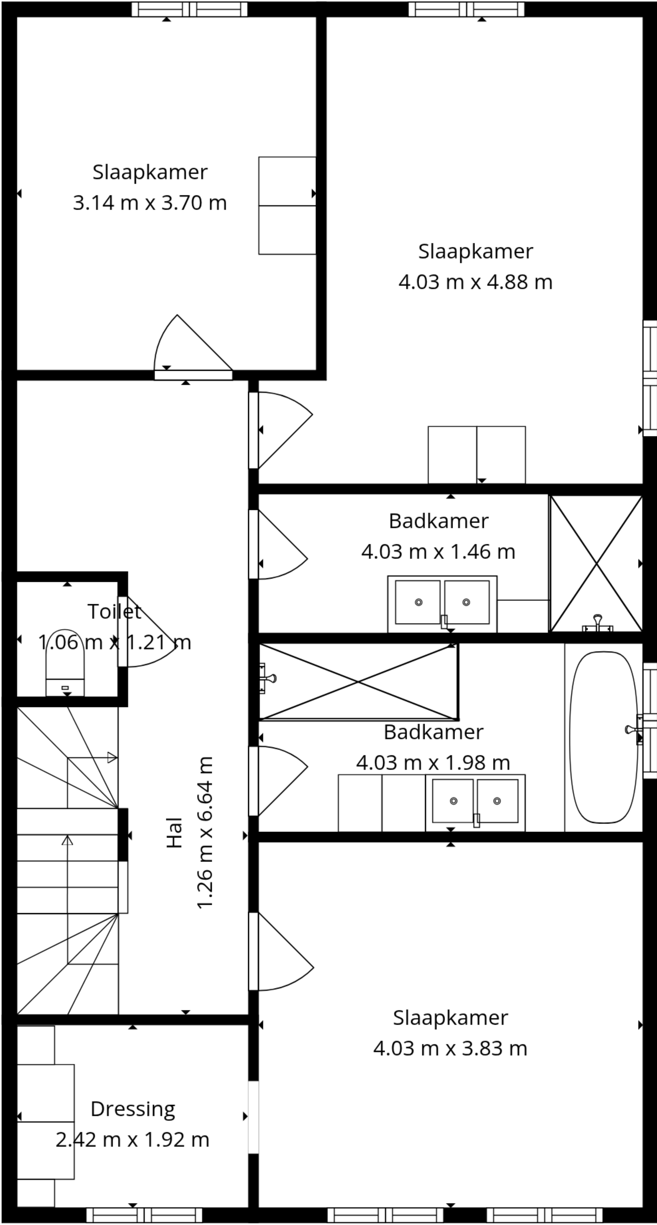
1e Verdieping
